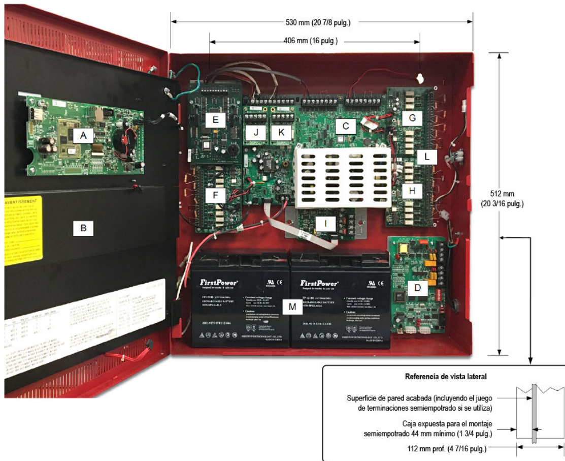
Figura 5: Referencia de montaje y ubicación de módulo de 4007ES
